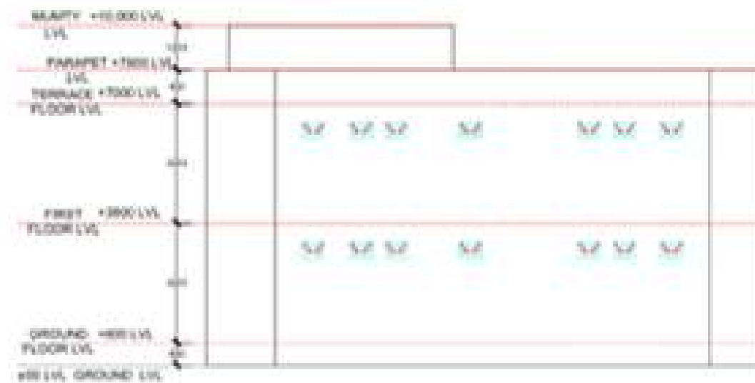
ELEVATION C-C'
